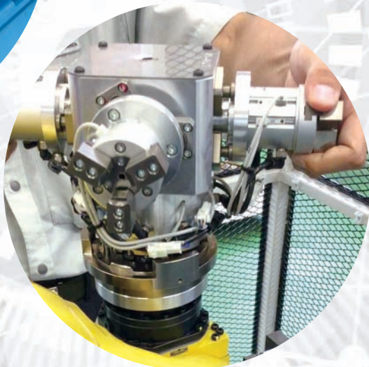
手動式ロボットハンドチェンジャー。 ボルト1本にて固定、 カービックカップリング方式
