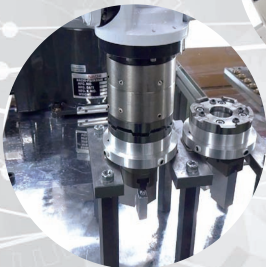
自社製ハンドチェンジャーでの 交換動作の様子
